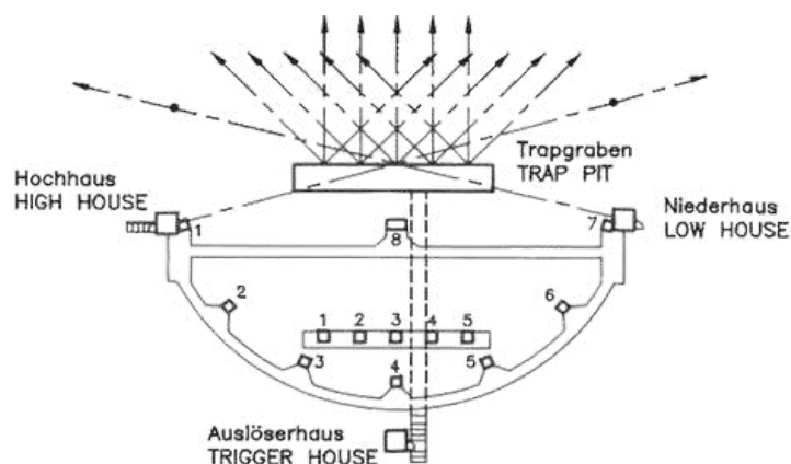
Trap- und Skeet- Schiessanlage kombiniert COMBINED TRAP AND SKEET RANGES
